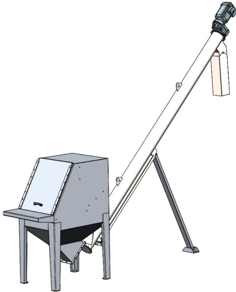
Рисунок 1. Общий вид растаривателя с ручной загрузкой
