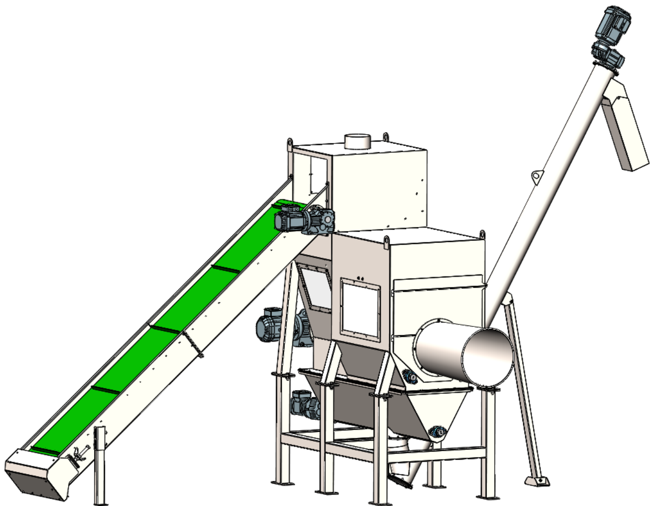
Рисунок 2. Общий вид растваривателя с автоматической загрузкой
